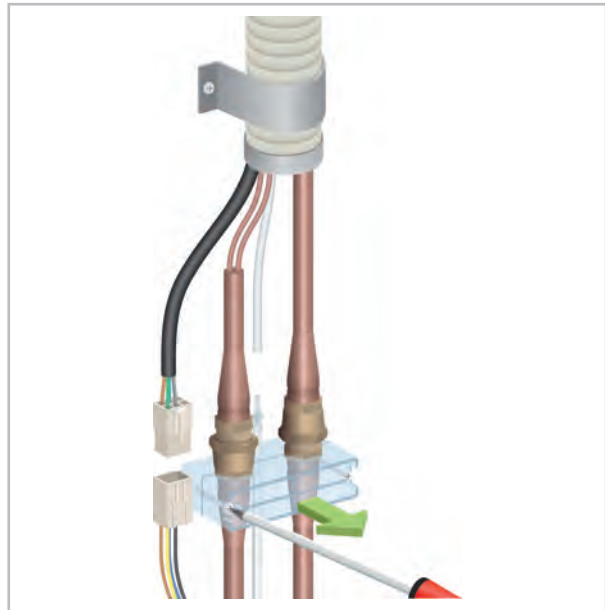
Abb. 16: Halterung entfernen
